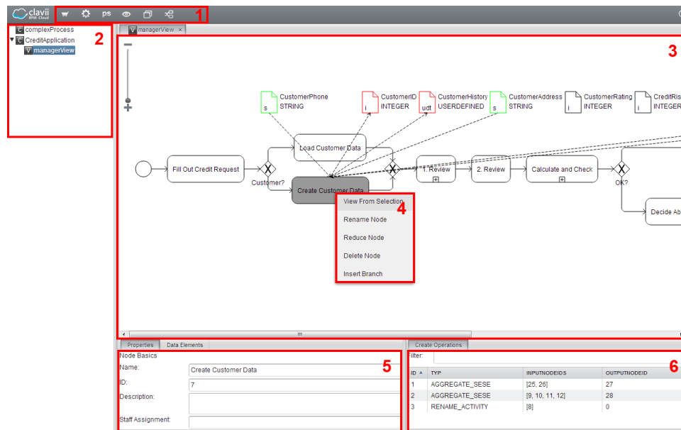
Abbildung 2.8: Webbasierte Benutzeroberfläche von proView.
