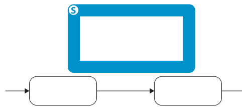
Abbildung 3.16: Datenelement einfügen.
