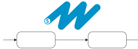
Abbildung 3.18: Rückgängig machen.
