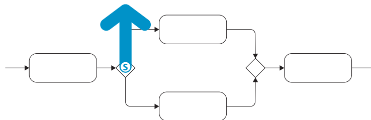
Abbildung 3.11: Verzweigung einfügen.
