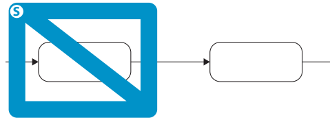
Abbildung 3.10: Element reduzieren.
