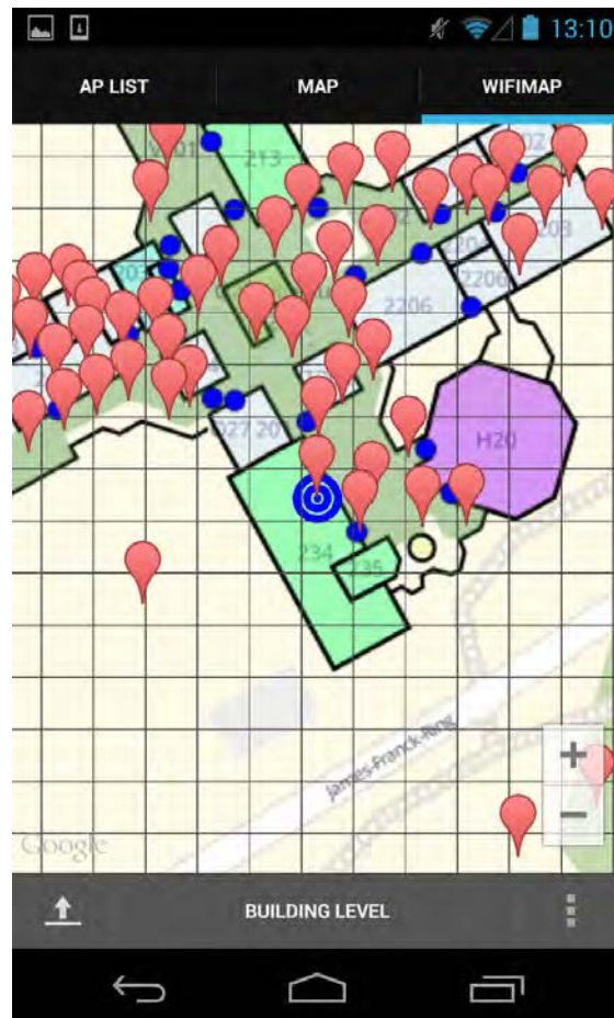
Abbildung 7.7: Wifimap zum anlegen von WiFi-Fingerabdrücken.
