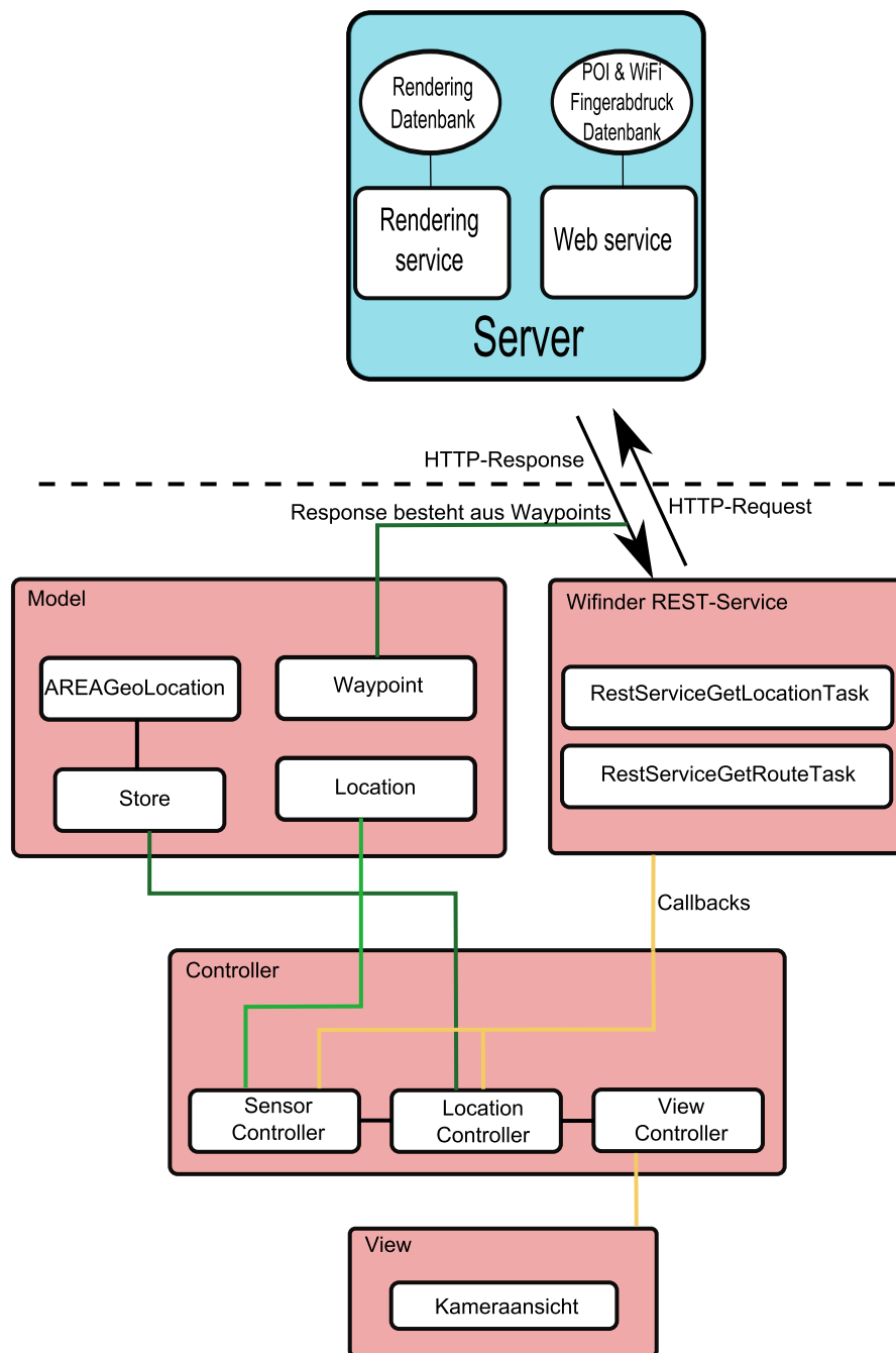
Abbildung 4.1: Überblick über die Architektur.
