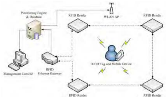
Abbildung 2.1: Schema des vorgeschlagenen RFID-Positionierungssystems. Vgl. [LCH11]
