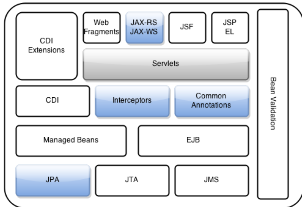
Abbildung 6.3: Java EE Komponenten nach [jav]
