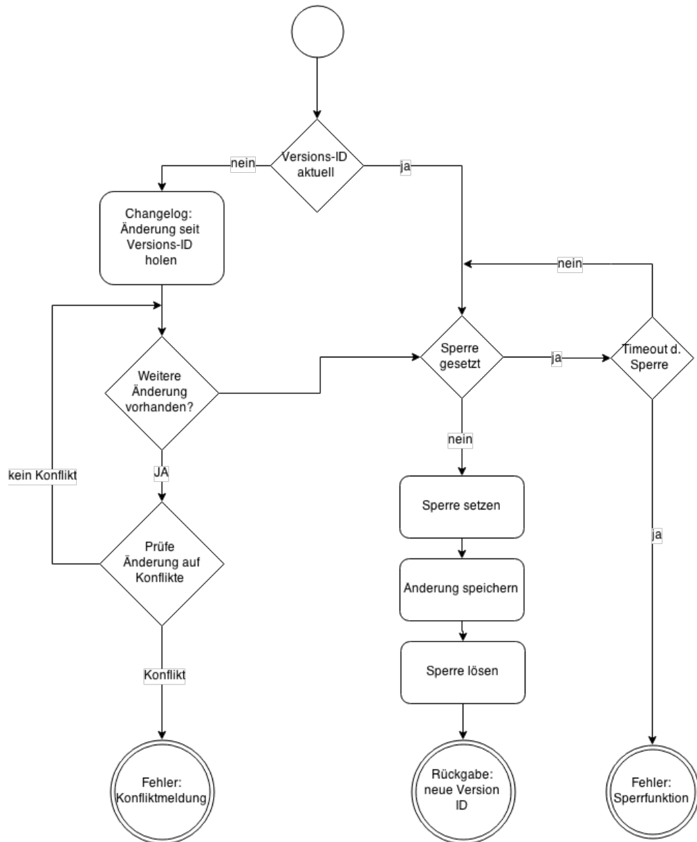
Abbildung 5.4: Konfliktlösung Serverseite 1
