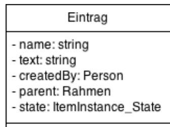
Abbildung 2.14: Datenmodell: Eintrag
