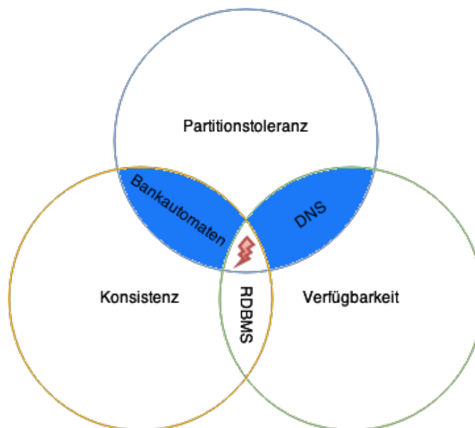
Abbildung 3.2: CAP-Theorem: Anwendungen
