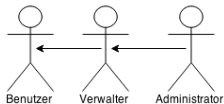
Abbildung 2.15: Nutzerrollen
