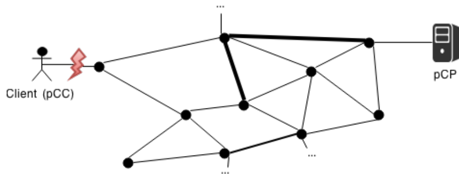
Abbildung 4.3: Inkonsistente Internetverbindung
