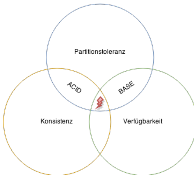
Abbildung 3.3: ACID und BASE innerhalb des CAP-Theorems
