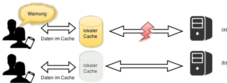
Abbildung 5.2: proCollab-Client: Cache auf der Clientseite
