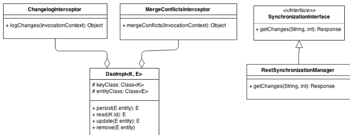
Abbildung 6.6: Beziehungen der Klassen
