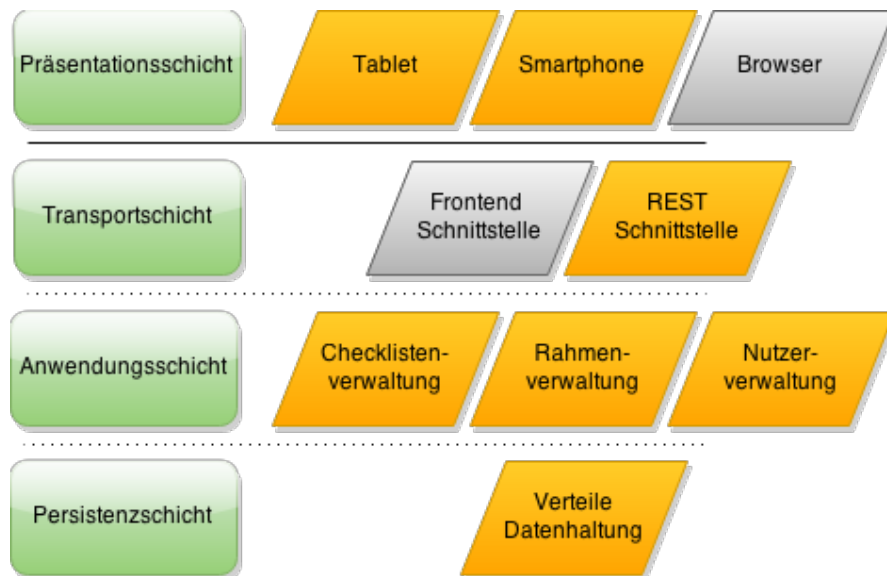
Abbildung 2.6: Applikationsschichten des pCP
