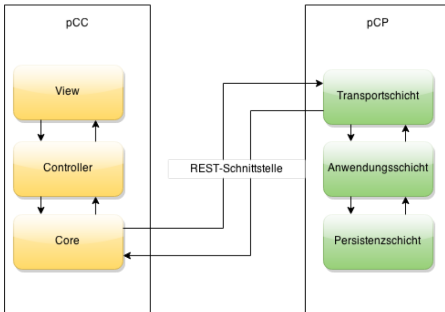
Abbildung 2.7: Applikationsschichten des pCC
