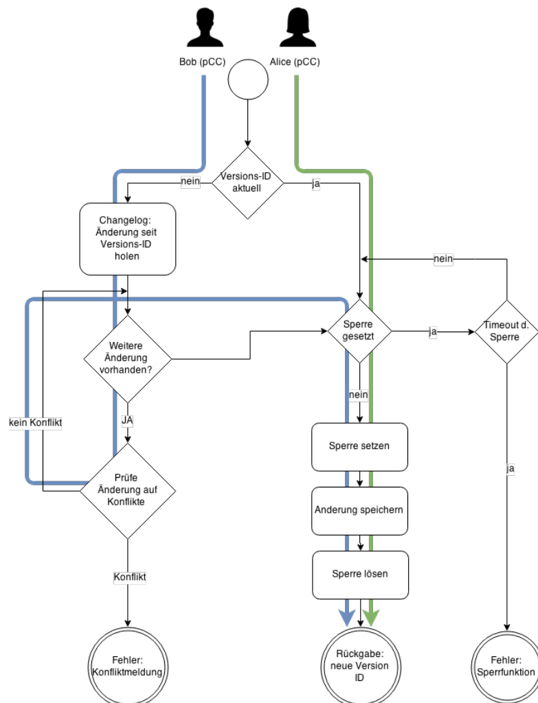
Abbildung 5.7: Konfliktlösung 1: pCP
