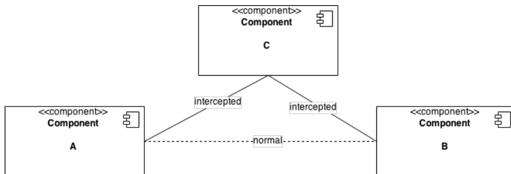
Abbildung 6.4: Interceptor Schema
