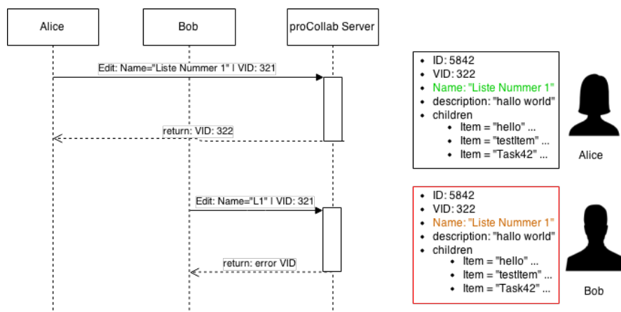
Abbildung 5.8: Konfliktlösung 2: pCC
