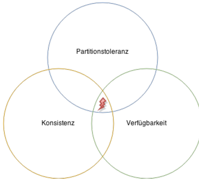
Abbildung 3.1: CAP-Theorem
