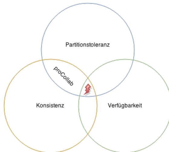
Abbildung 4.13: CAP-Theorem: proCollab
