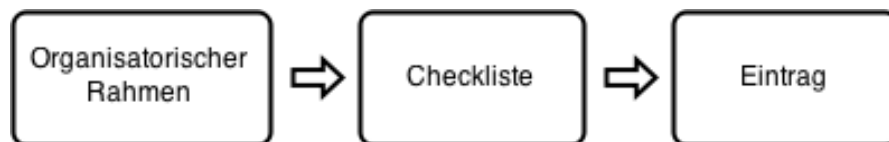
Abbildung 2.8: Hierarchisches Datenbankmodell
