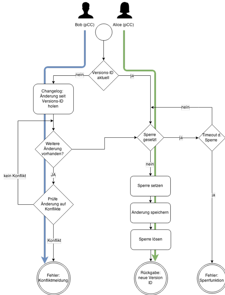
Abbildung 5.9: Konfliktlösung 2: pCP
