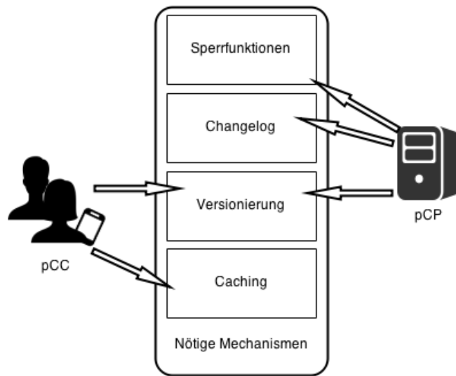
Abbildung 5.1: Benötigte Mechanismen
