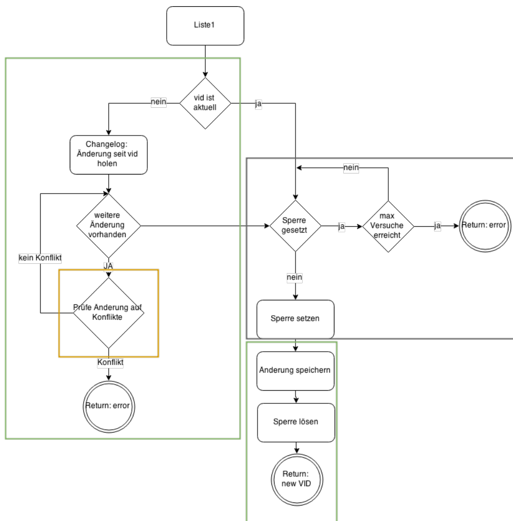
Abbildung 6.5: Konfliktlösung Implementierung
