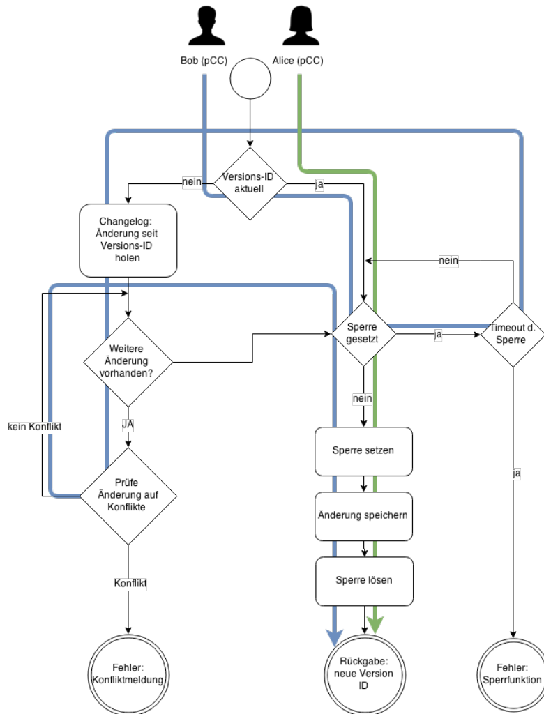
Abbildung 5.10: Konfliktlösung 2: Server
