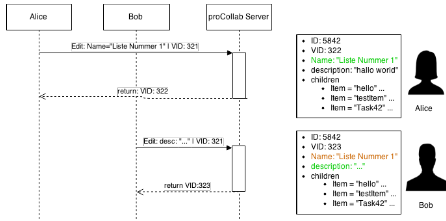
Abbildung 5.6: Konfliktlösung 1: pCC
