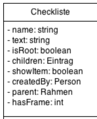
Abbildung 2.12: Datenmodell:Checkliste
