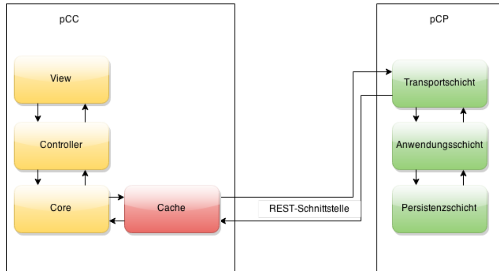
Abbildung 6.7: pCC: Cache
