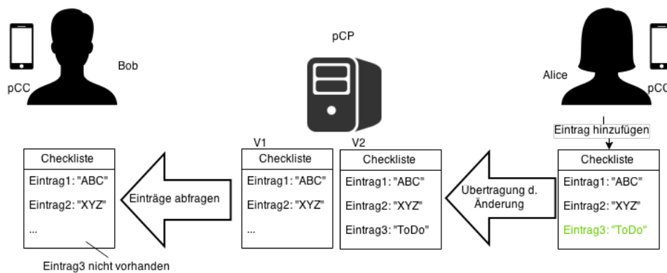
Abbildung 4.8: AF3: Phantomproblem
