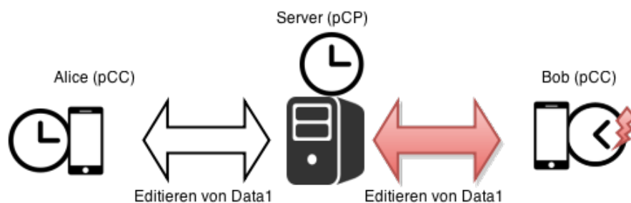
Abbildung 4.4: Zeitproblem
