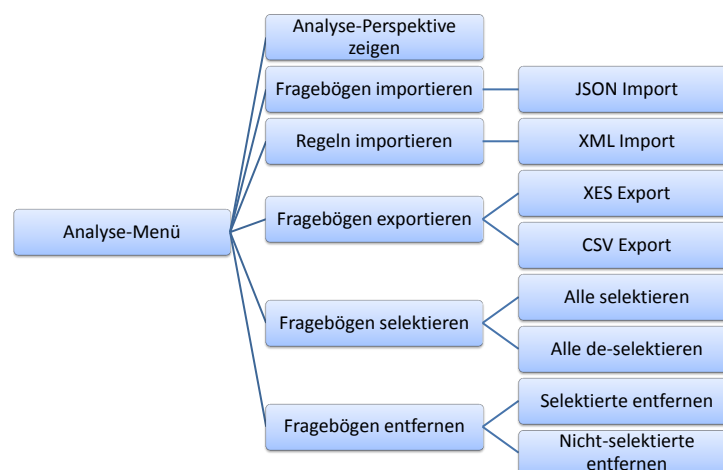
Abbildung 6.3: Menübaum Analysekomponente
