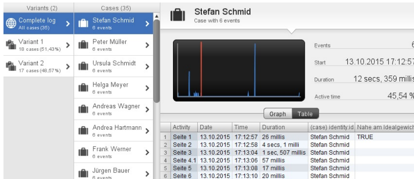
Abbildung 5.9: Disco Cases
