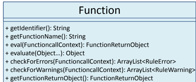
Abbildung 5.3: Function Interface [5]
