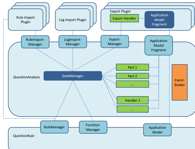
Abbildung 5.1: Architektur QuestionAnalysis
