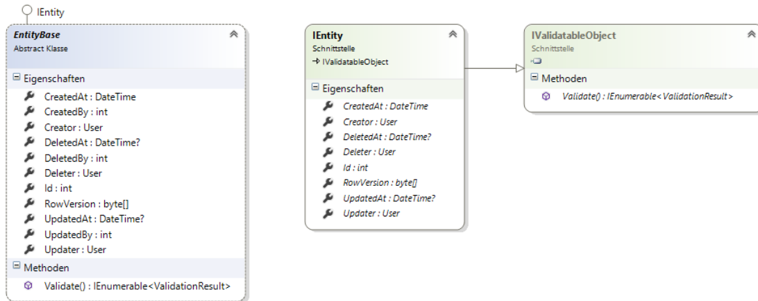
Abbildung 6.2: Abstrakte Basisklasse für Entitäten als Klassendiagramm (Visual Studio Export)
