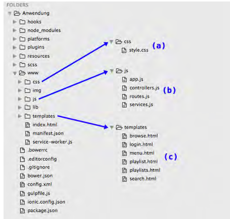
Abbildung 4.6: Die Ordnerstruktur eines Ionic-Projektes
