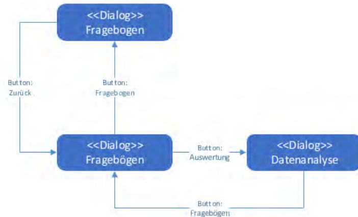
Abbildung 5.5.: Dialogstruktur Fragebögen
