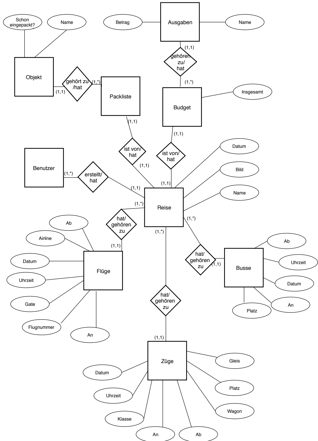
Abbildung 4.1: Entity-Relationship-Diagramm zur Anwendung. Die Entitäten Reise, Busse, Flüge, Züge, Benutzer, Budget, Ausgaben und Objekt werden zueinander in Relation gesetzt und die jeweiligen Attribute zugeordnet.
