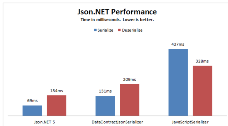
Abbildung 2.2: Performancevergleich von Json.Net mit DataContractJsonSerializer und JavaScriptSerializer [5]
