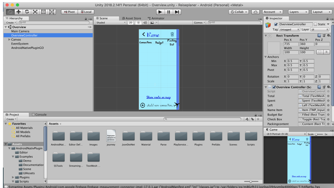
Abbildung 2.1: Der grundsätzliche Aufbau von Unity in Scene, Inspector, Project, Game und der Hierarchy
