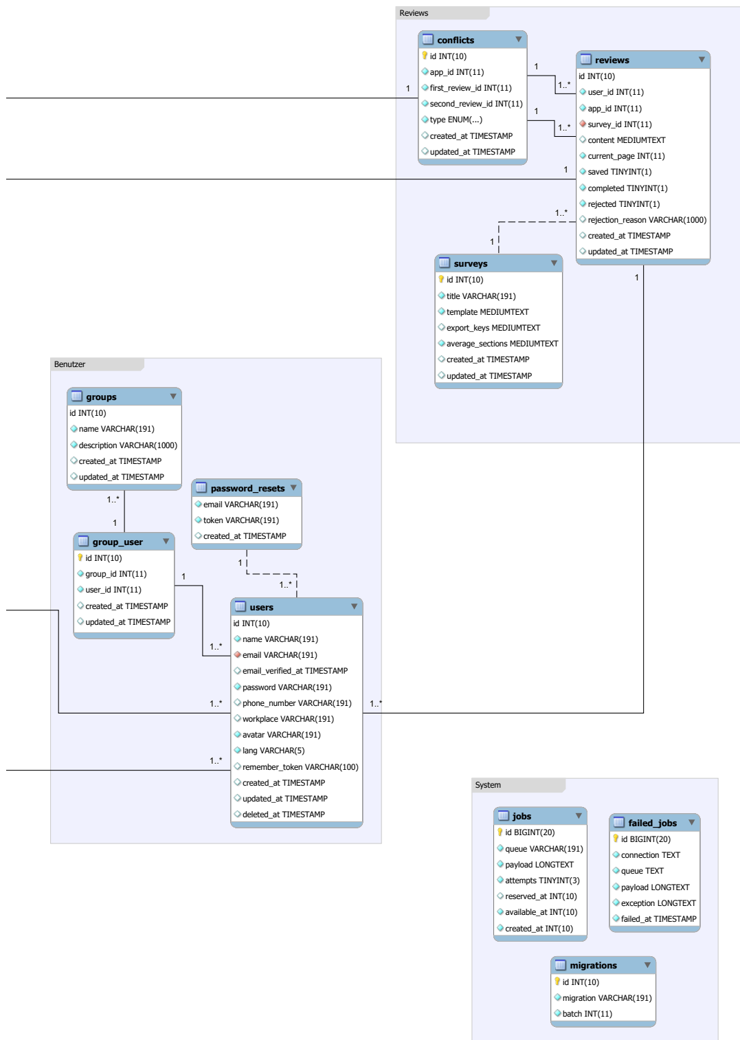
Abbildung 4.8: Das Schema der Systemdatenbank
