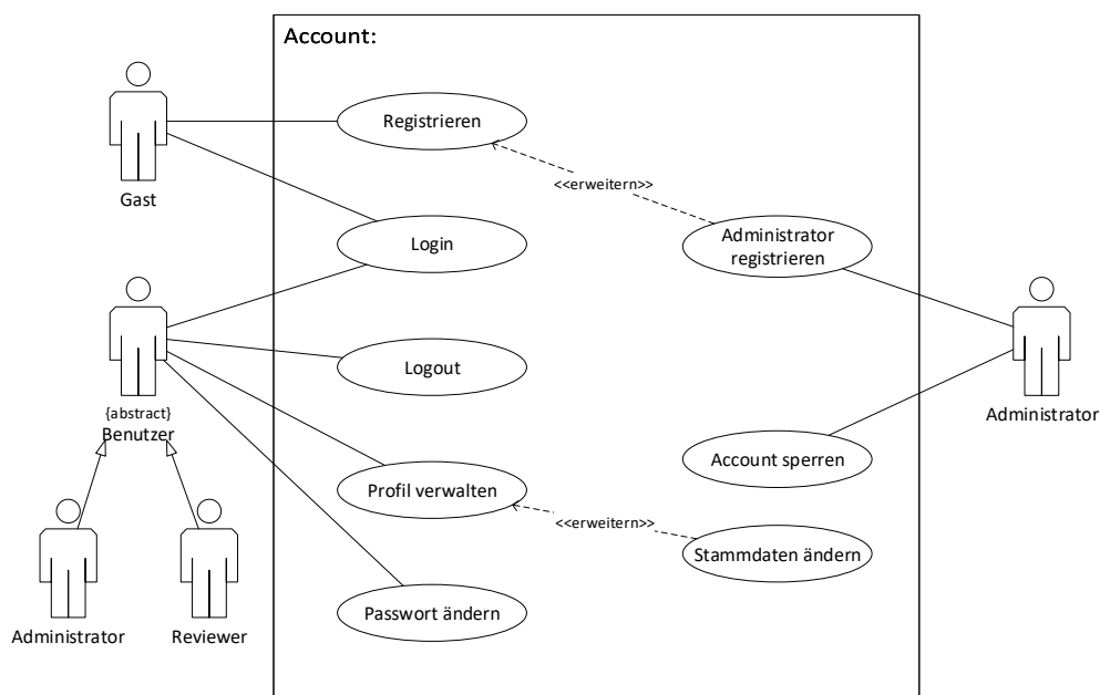
Abbildung 3.1: Anwendungsfalldiagramm für das Account-Modul
