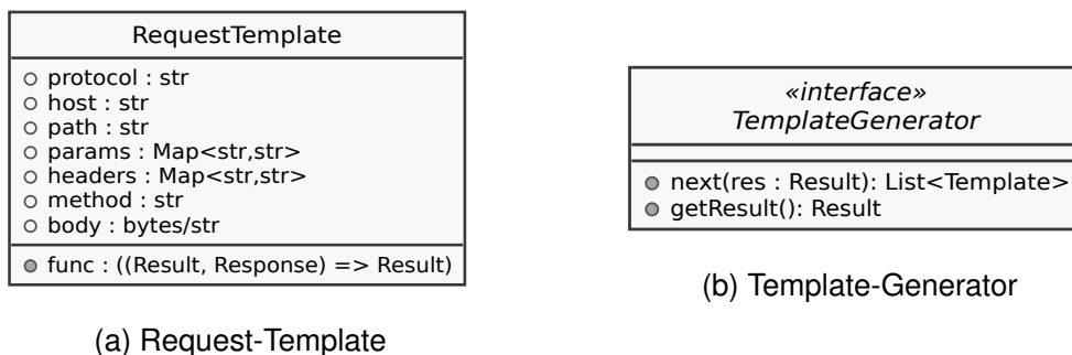
Abbildung 4.4: Konzept von Request-Templates
