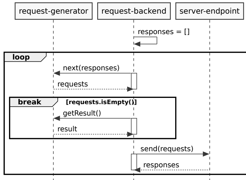
Abbildung 4.3: RequestGenerator-Datenfluss
