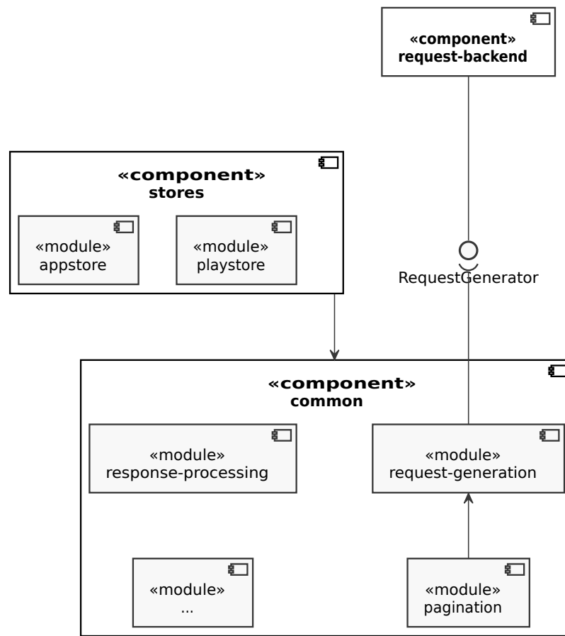
Abbildung 4.1: Komponentendiagramm für den Scraper-Kern
