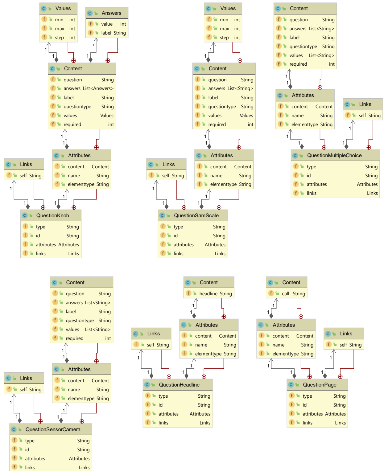
Abbildung 10: UML-Klassendiagramm Questions Teil 1
