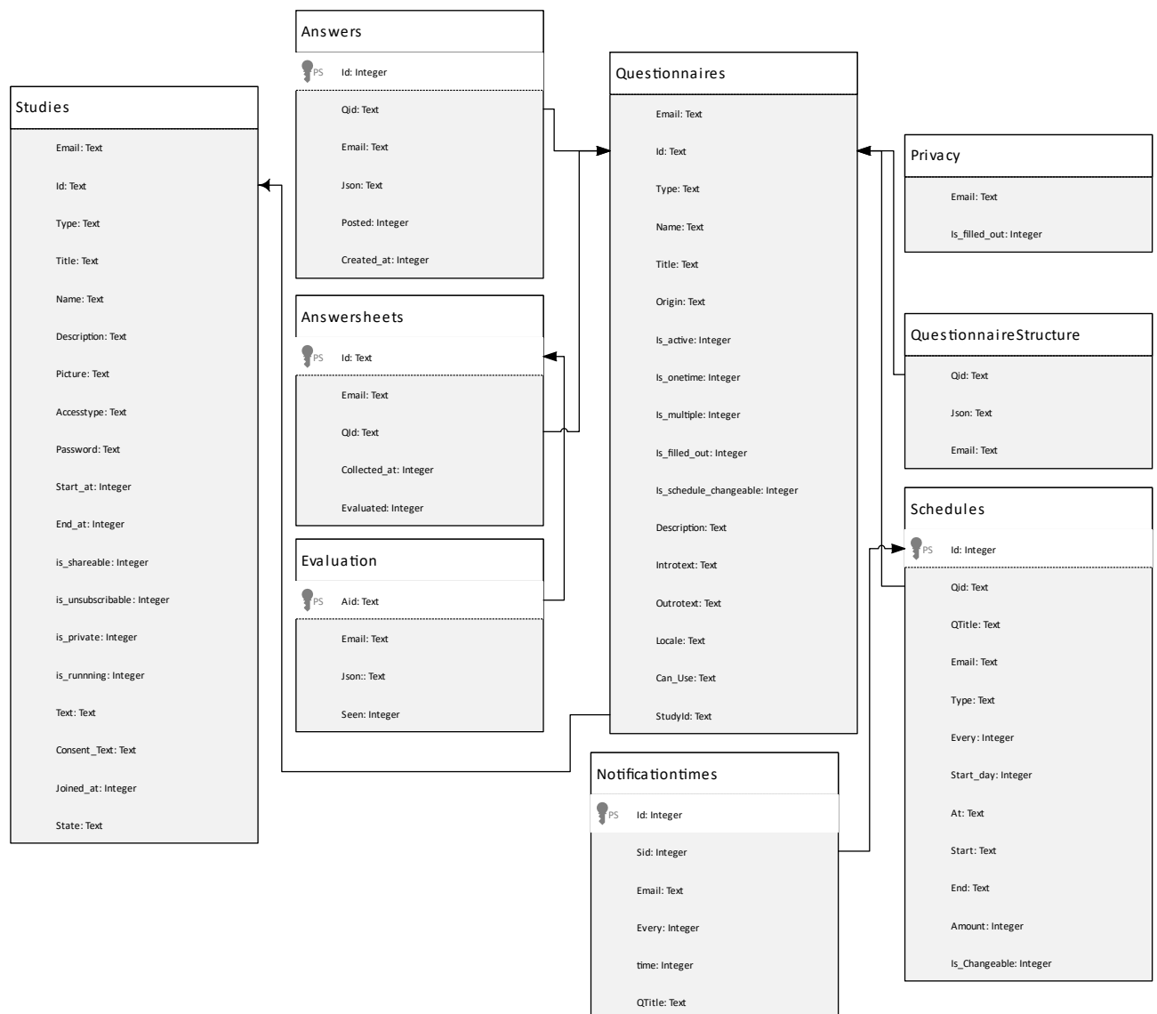
Abbildung 6: UML-Datenbankdiagramm Lokale Datenbank
