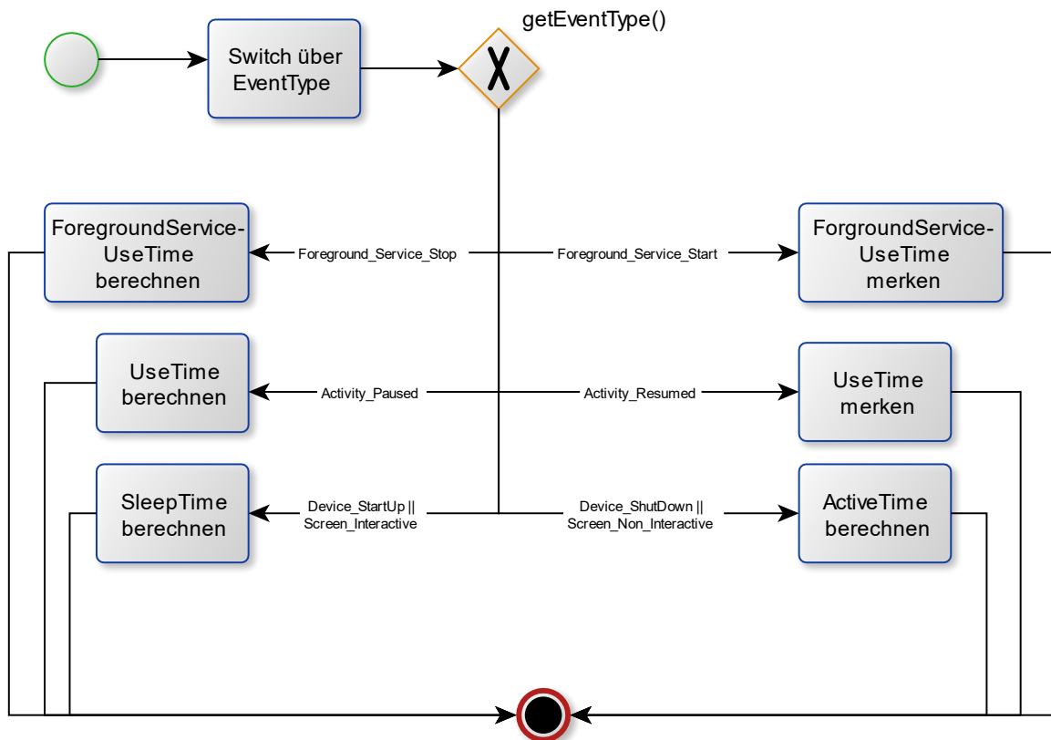
Abbildung 18: Implementierung EventTypes
