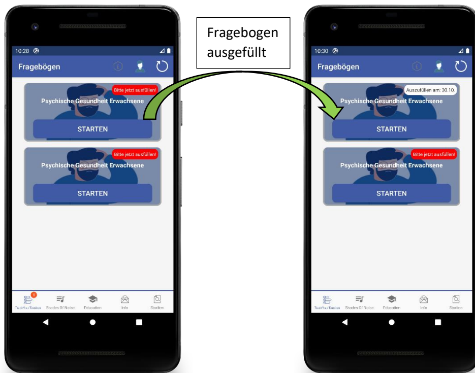
Abbildung 21: Fragebögen-Ansicht
