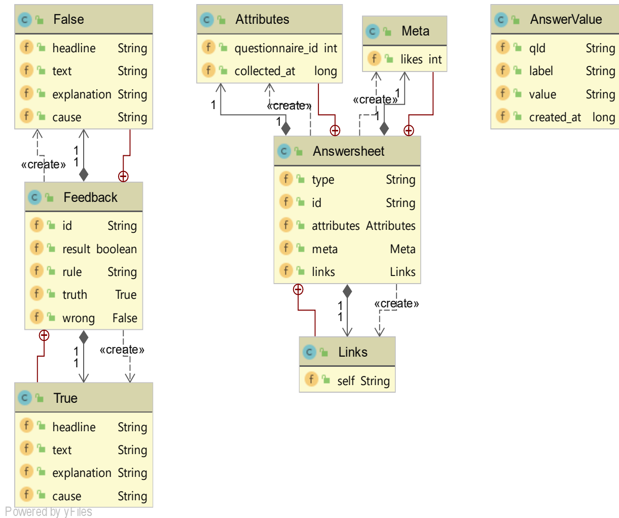
Abbildung 12: UML-Klassendiagramm Feedback
