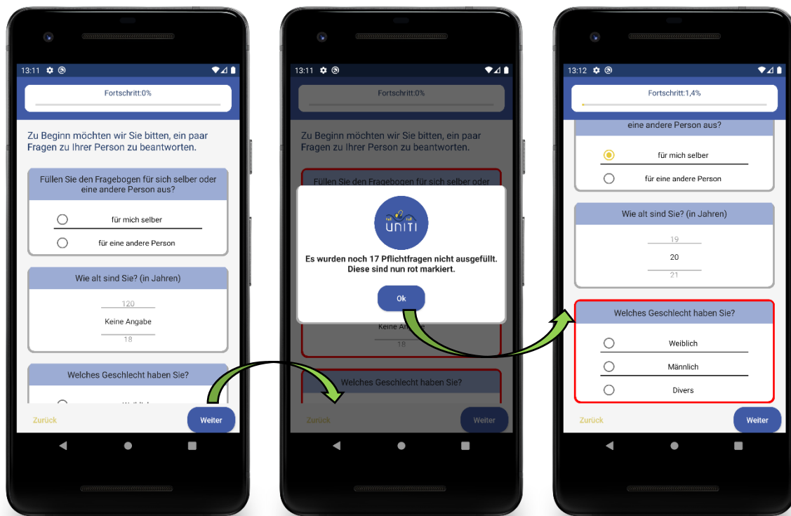
Abbildung 25: Fragebogenstruktur Fehlermeldung
