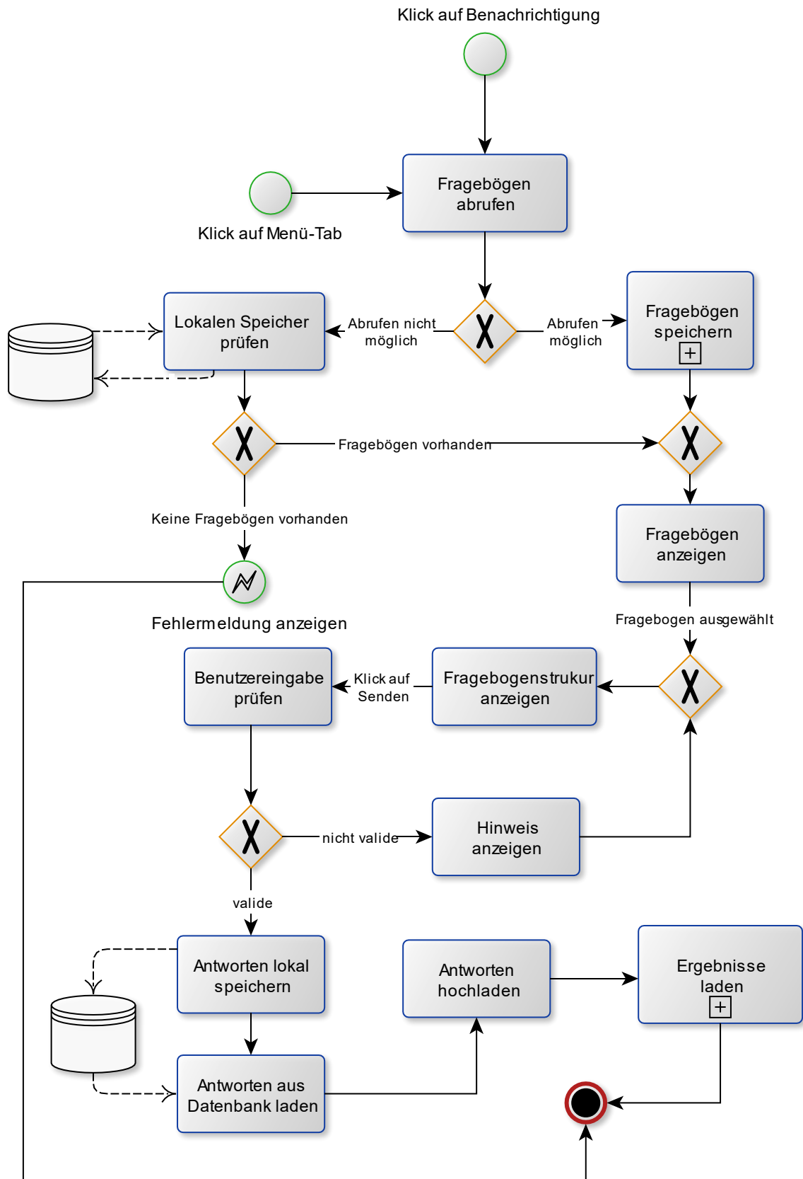
Abbildung 2: Prozessablauf-Diagramm Fragebogenmodul
