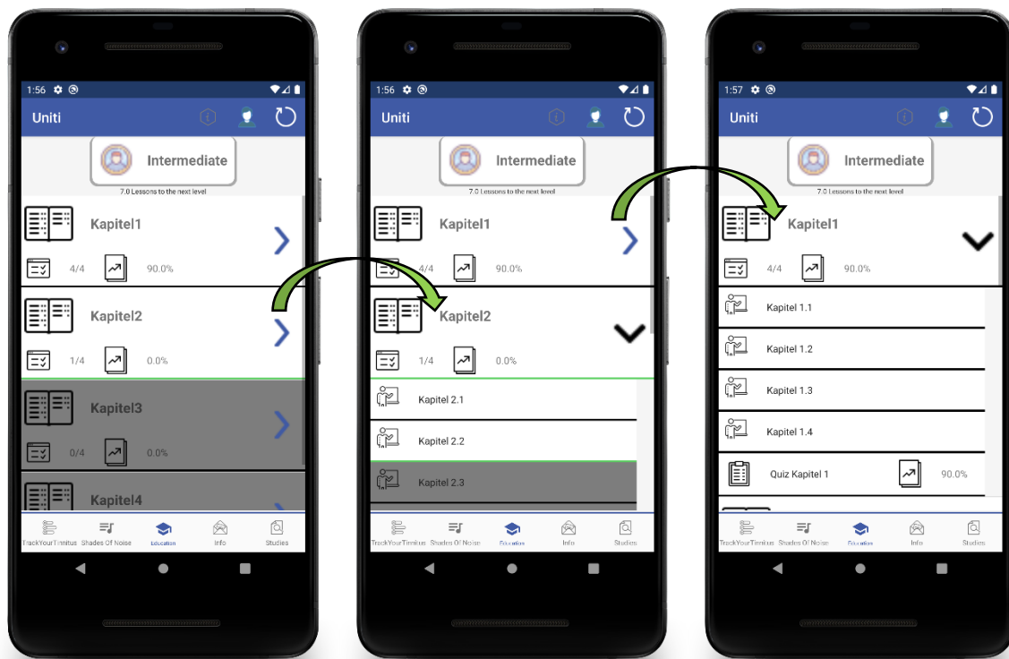
Abbildung 19: Kapitelstruktur
