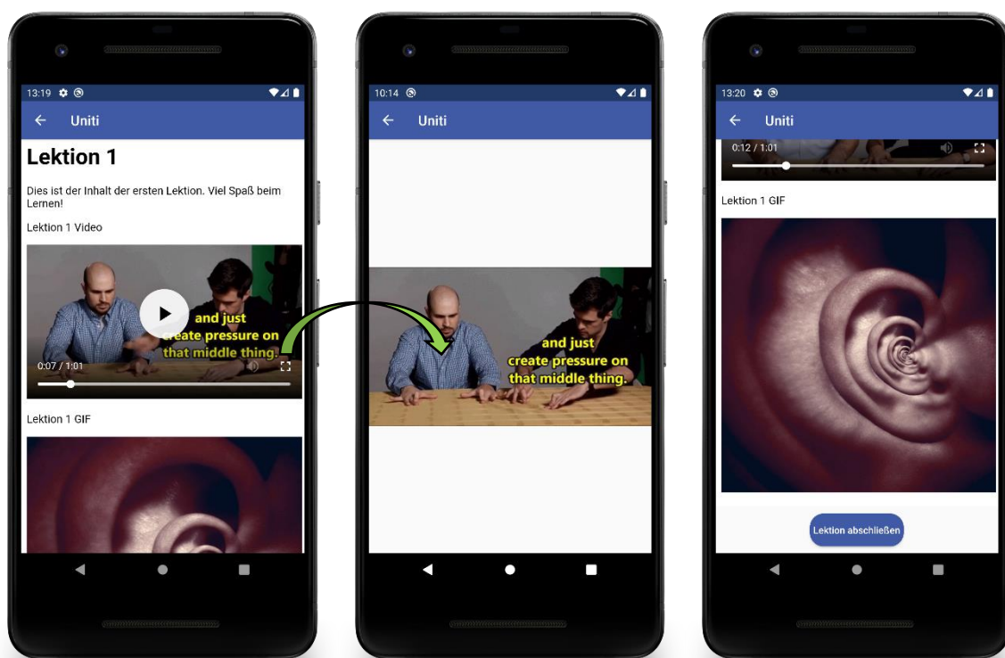
Abbildung 20: Unterkapitel
