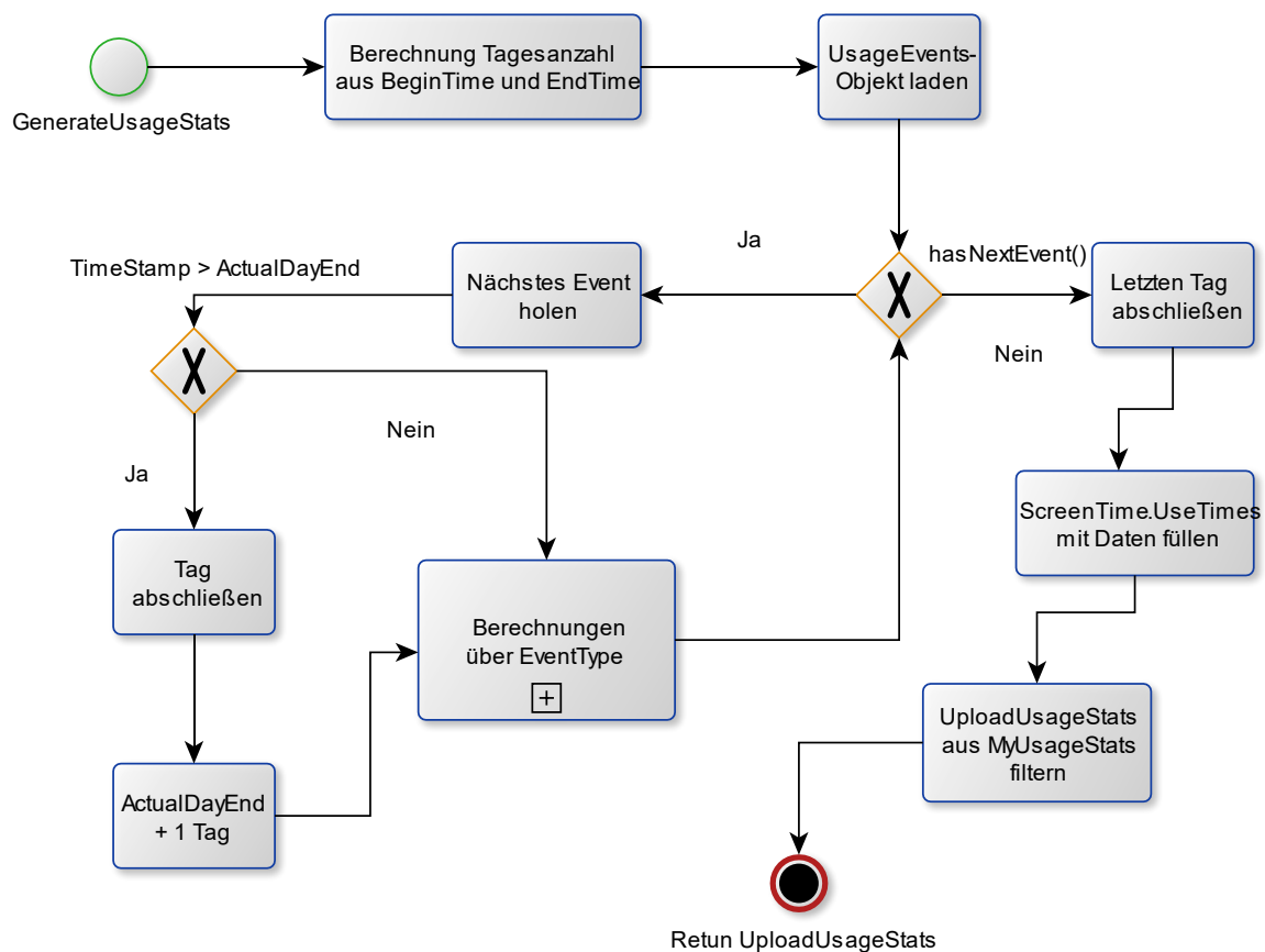
Abbildung 17: Implementierung UsageStats
