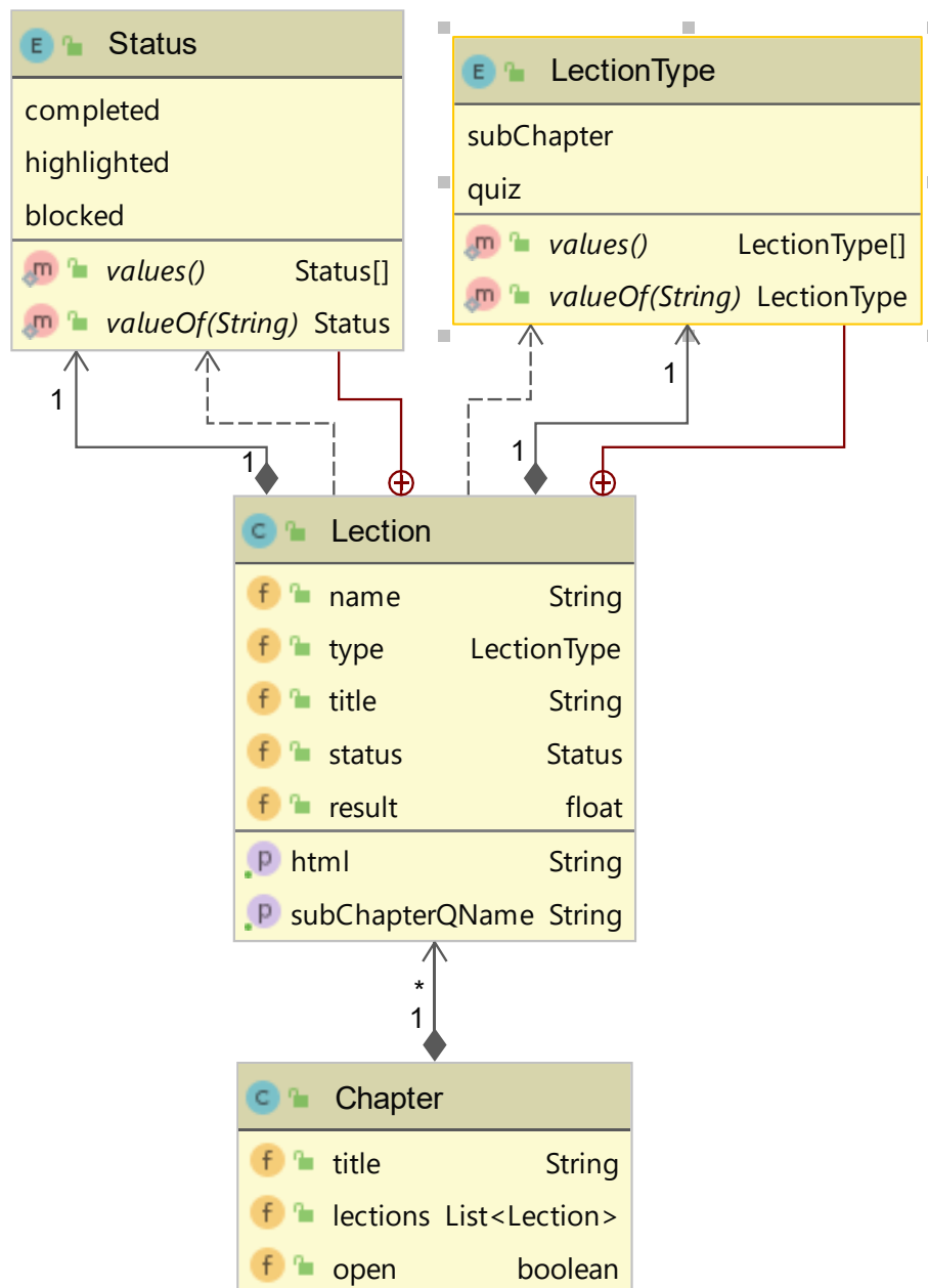
Abbildung 7: UML-Klassendiagramm Kapitel und Lektionen
