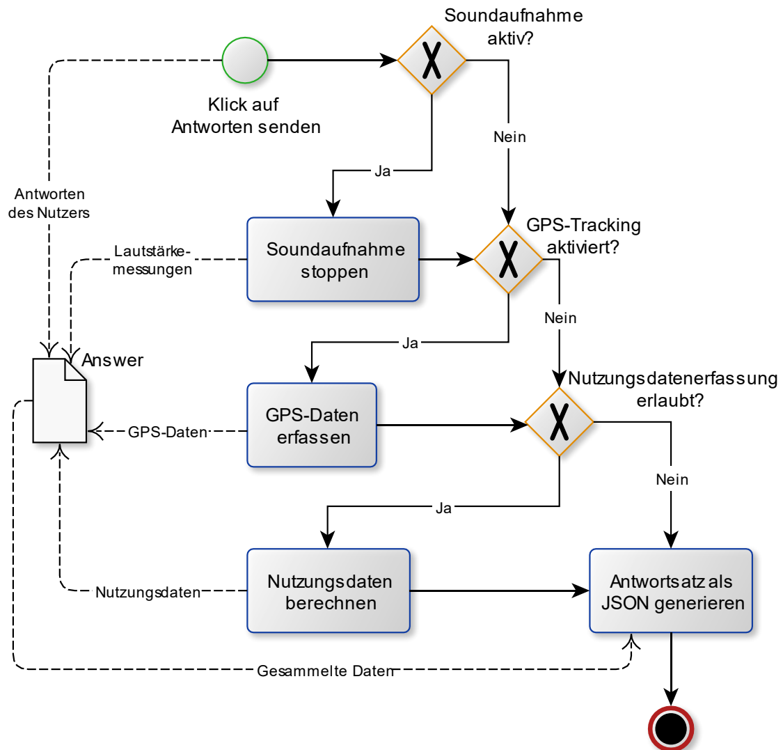
Abbildung 5: Prozessablauf-Diagramm Antwortsatz erstellen
