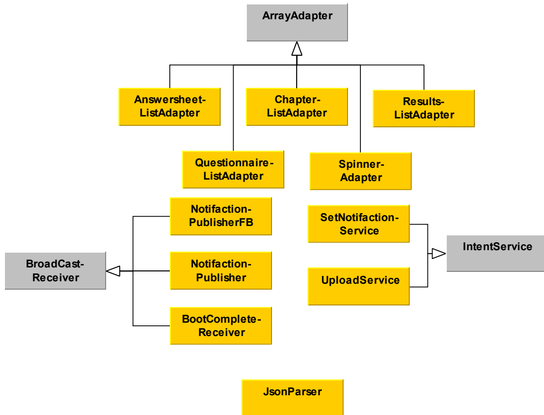
Abbildung 15: UML-Klassendiagramm ListAdapter, Receiver und Services
