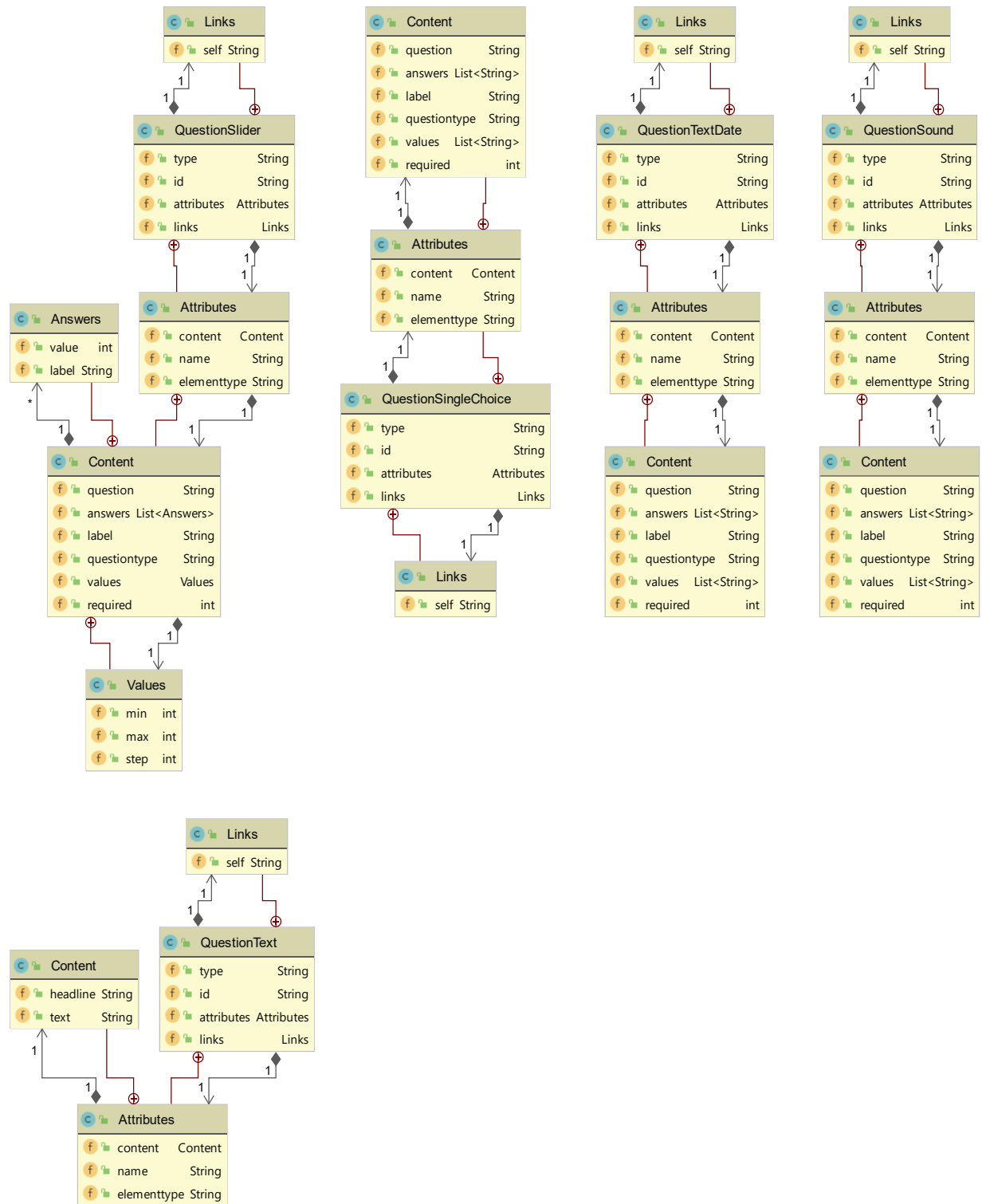
Abbildung 11: UML-Klassendiagramm Questions Teil 2
