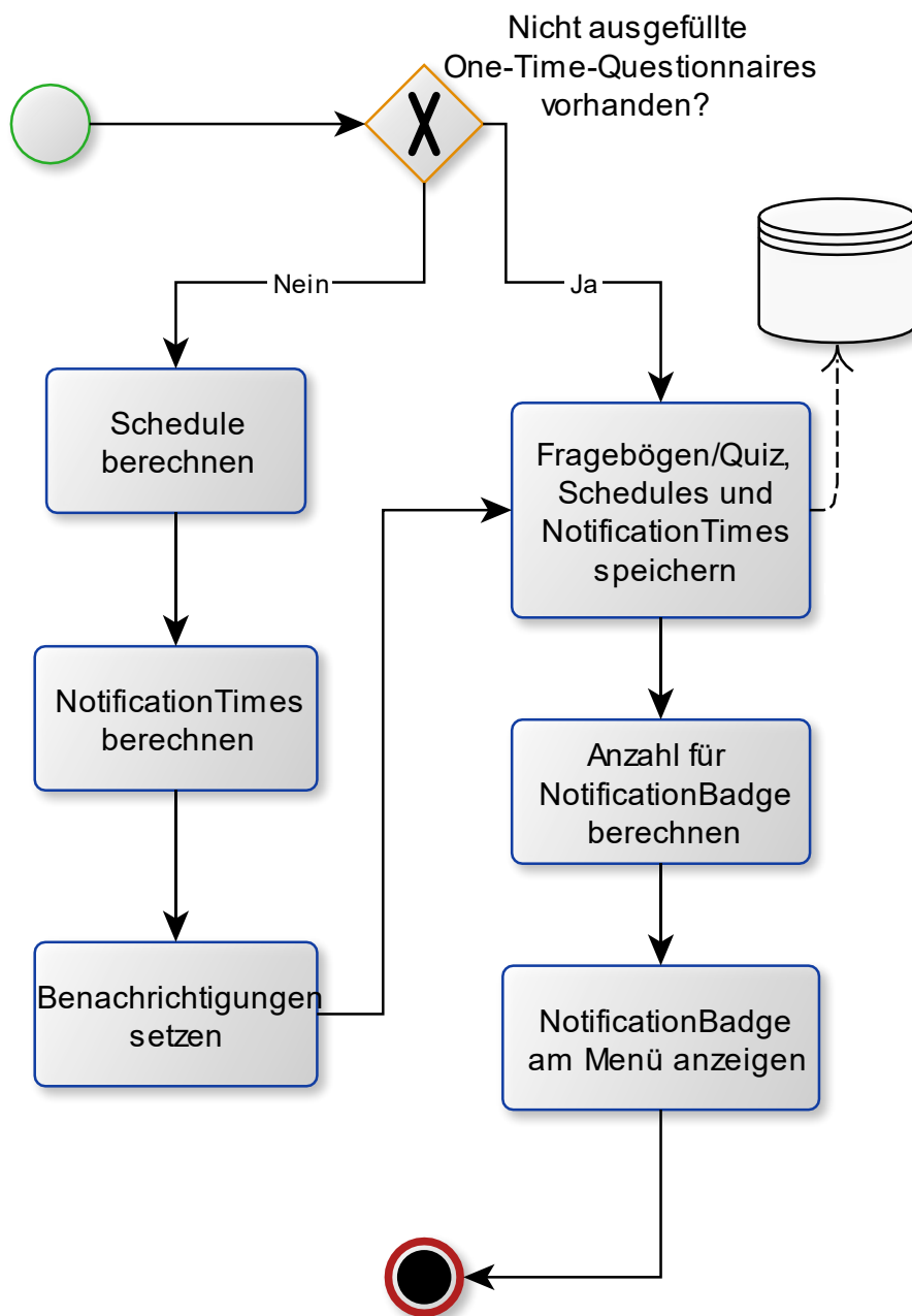
Abbildung 4: Prozessablauf-Diagramm Fragebögen speichern
