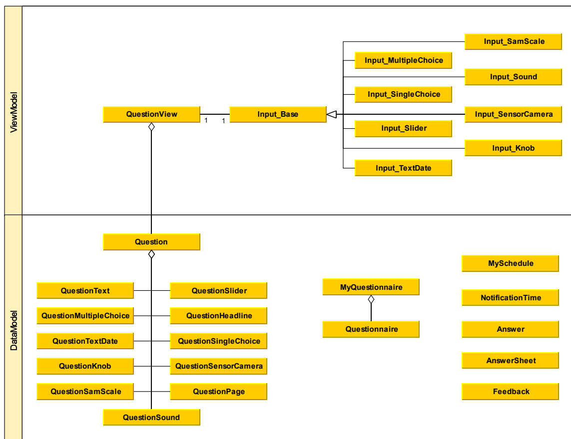
Abbildung 14: UML-Klassendiagramm ViewModel und DataModel
