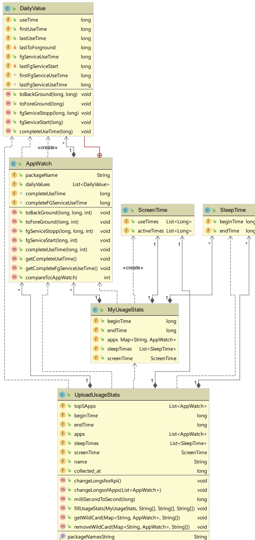
Abbildung 8: UML-Klassendiagramm UsageStats
