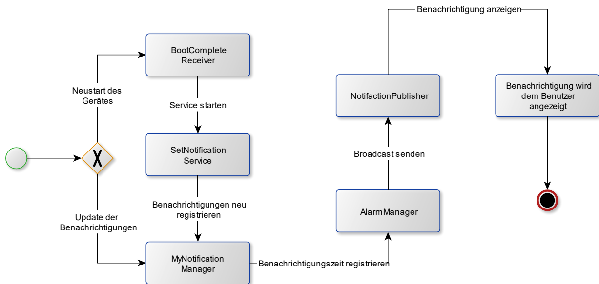
Abbildung 16: Ablaufskizzierung Benachrichtigungen
