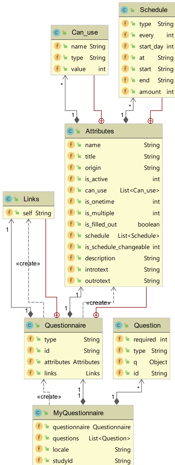
Abbildung 9: UML-Klassendiagramm Questionnaire
