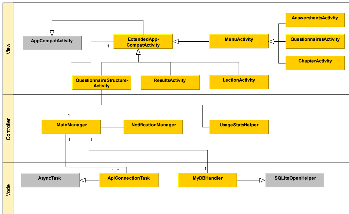
Abbildung 13: UML-Klassendiagramm Model-View-Controller
