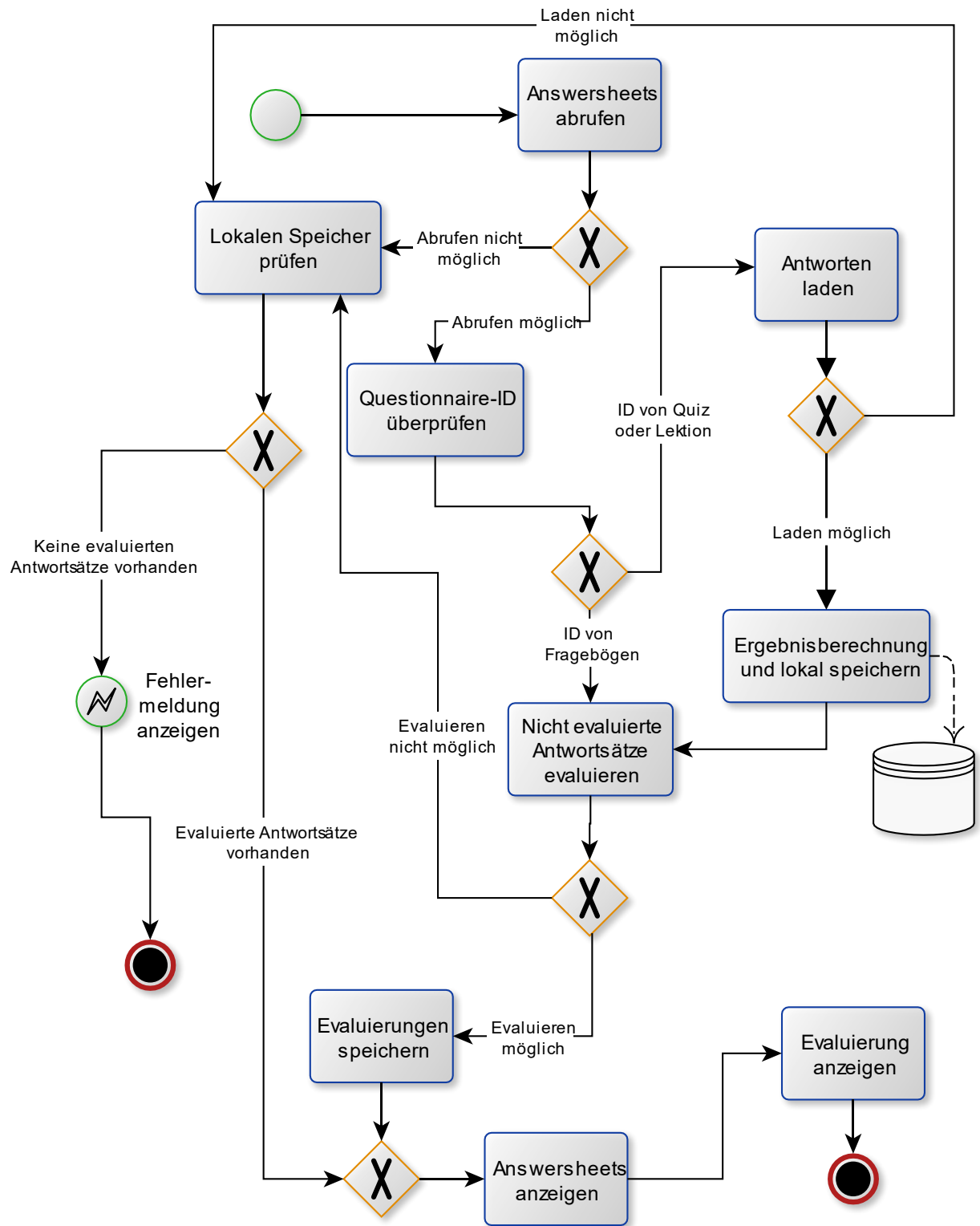
Abbildung 3: Prozessablauf-Diagramm Feedback
