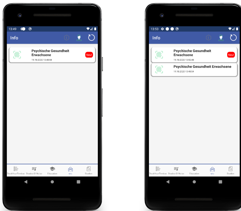
Abbildung 26: Antwortsätze
