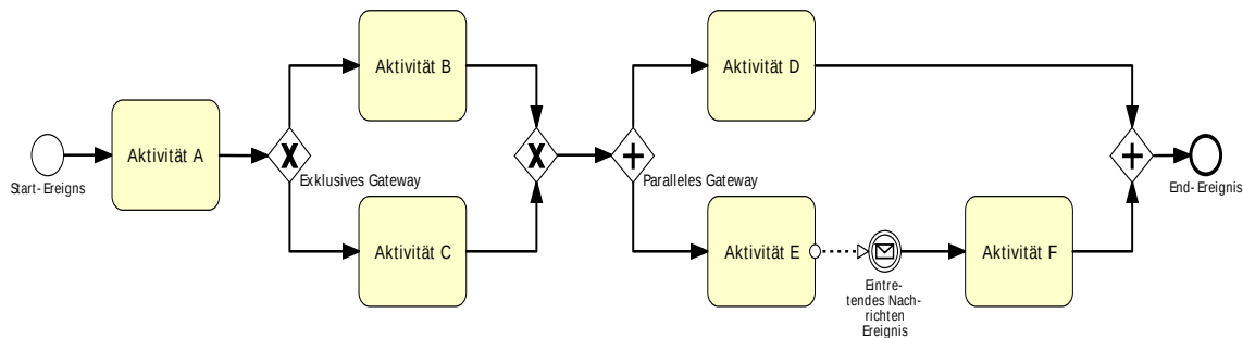
Abbildung 2.1: Beispielsprozess P
