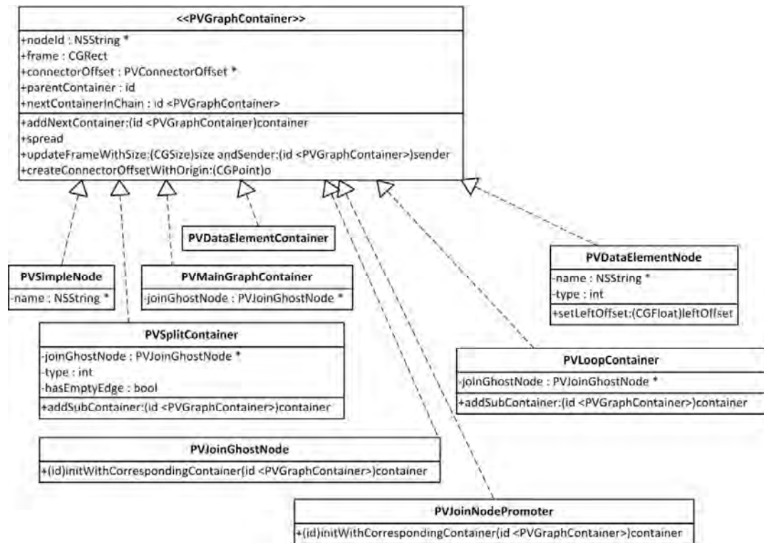
Abbildung 43: PVGraphContainer und implementierende Klassen
