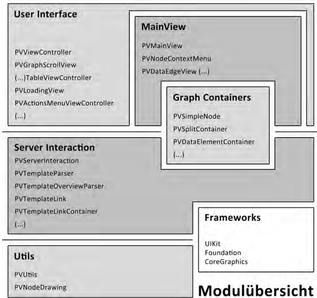
Abbildung 42: Übersicht über alle Programm-Module in proViewMobile
