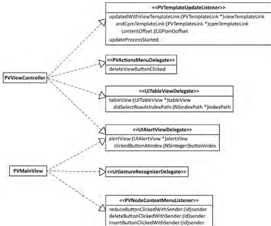
Abbildung 44: PVViewController und PVMainView als Delegates und Listener
