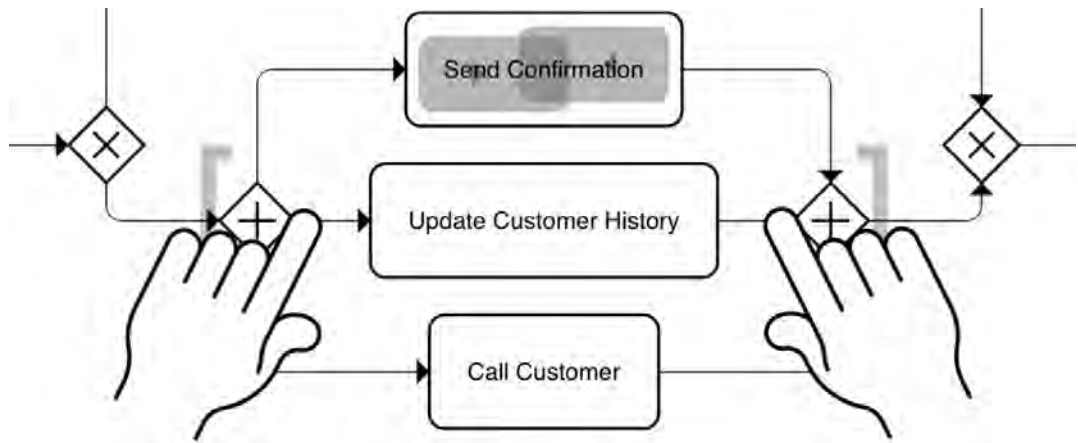
Abbildung 40: Aggregations-Geste
